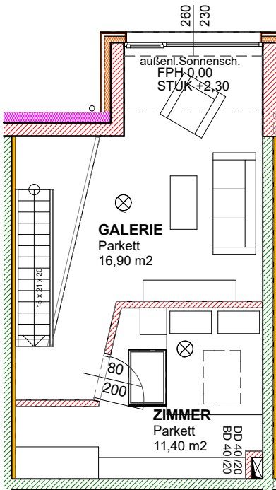
OBERGESCHOSS, M 1:100
