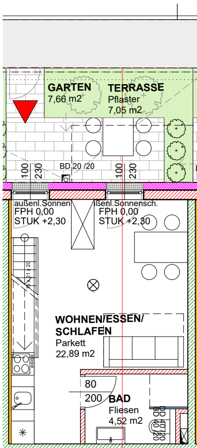
ERDGESCHOSS, M 1:100
