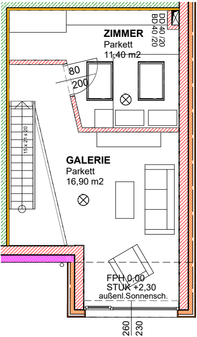
OBERGESCHOSS, M 1:100
