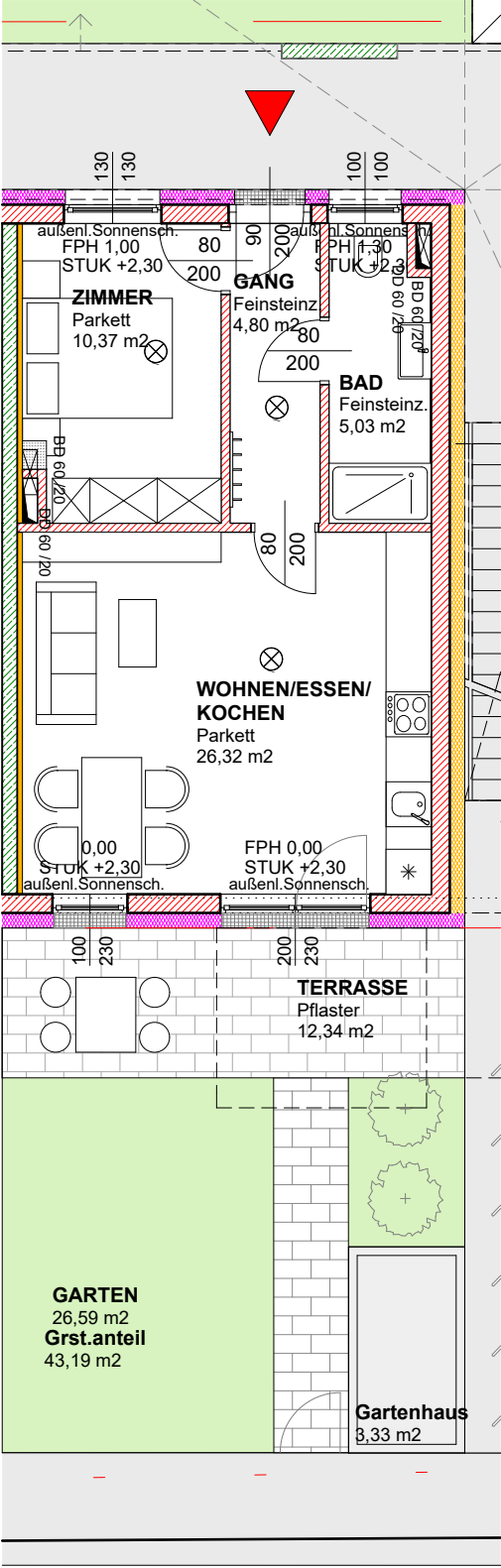
ERDGESCHOSS, M 1:100
