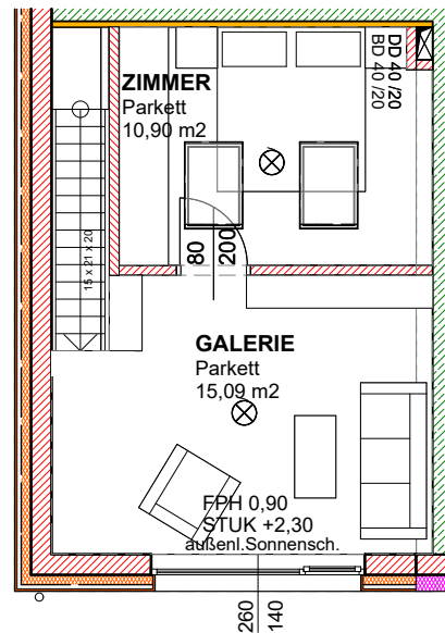
OBERGESCHOSS, M 1:100
